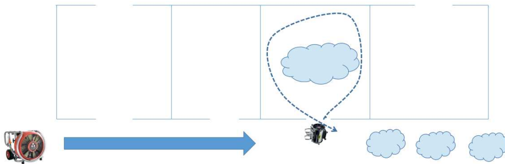
Illustration n°10 : Principe d'utilisation de ventilateurs dans une structure complexe disposant de locaux borgnes
